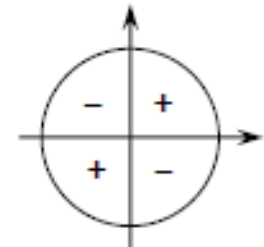
\operatorname{tg} t, \operatorname{ctg} t
