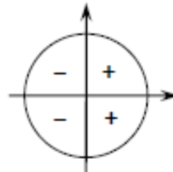
\cos t
